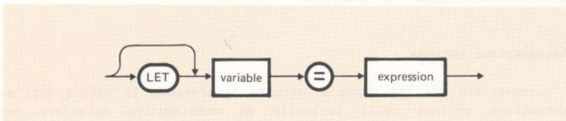
Figura 5-2 Istruzione LET
